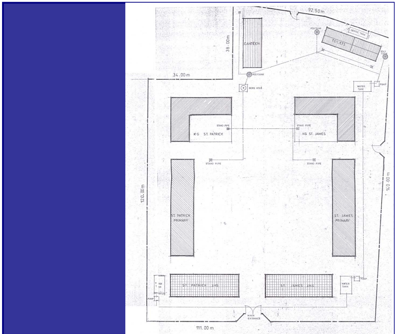
Plano general del proyecto Derribo y Reconstrucción de las Escuelas de St. James y St. Patrick. Sunyani, Ghana.
